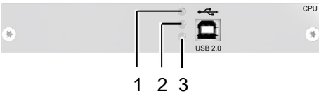
Fig. 42 Interface side add-on module USB 2.0 – Status LEDs L-/R474-BXE2
