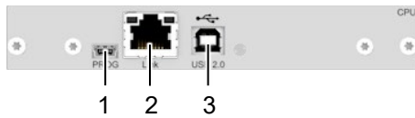
Fig. 34 Interface side L-/R474-BXUC
