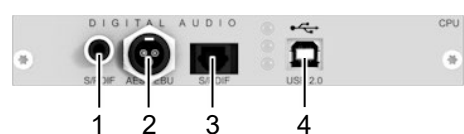
Fig. 25 Interface side L-/R474-BDE2
